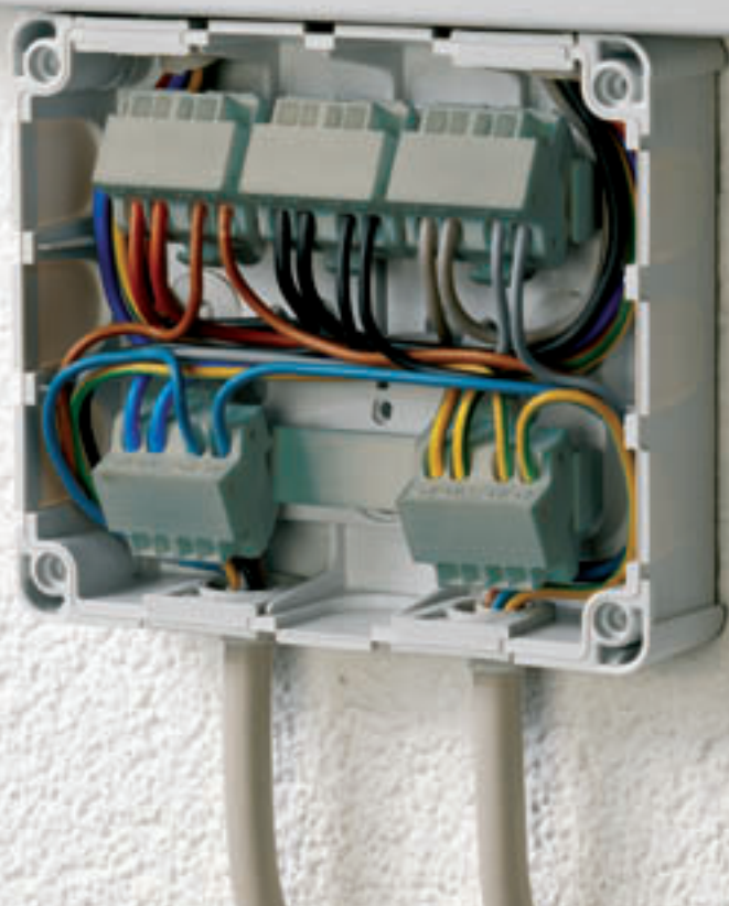
Надежные втычные клеммы FIXCONNECT в кабельных Коробках
