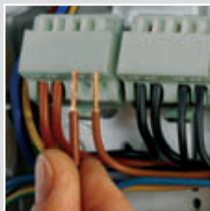
Соединение кабеля различного типа (многожильного и литого) в одном клеммнике
