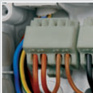
Надежные втычные клеммы FIXCONNECT в кабельных Коробках
